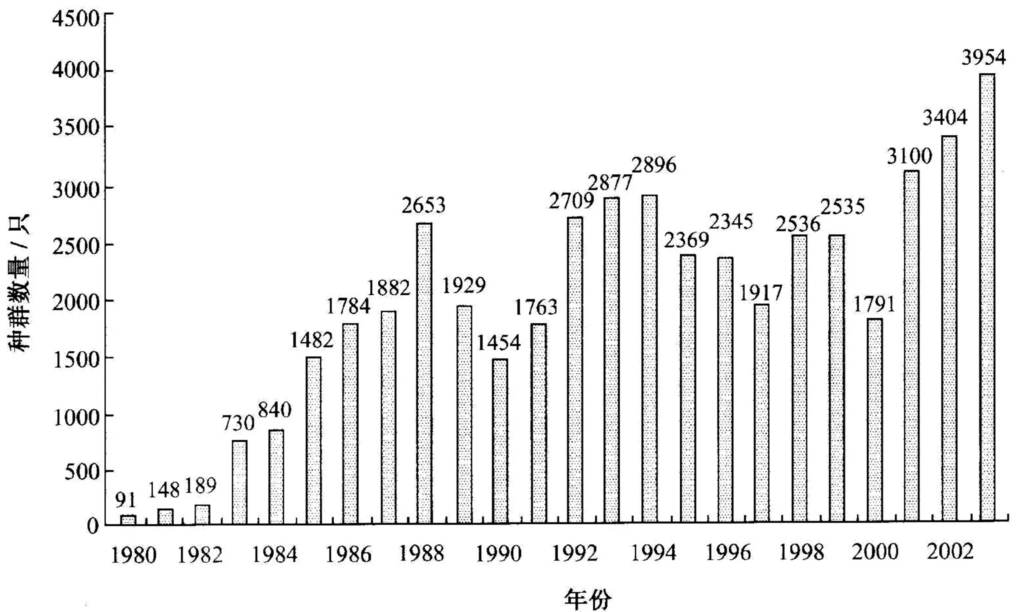
图 11 鄱阳湖自然保护区 1980—2003 年冬季白鹤的种群数量
